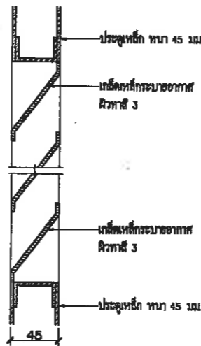
แบบขยายช่องแสงติดตาย มาตราส่วน 1: 2.5 AT A1 1: 5 AT A3 5
