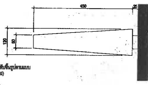
แปลน SCALE 1:5 AT A1 1:10 AT A3
