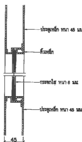
แบบขยายช่องแสงติดตาย มาตราส่วน 1: 2.5 AT A1 1: 5 AT A3 3
